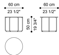
LOW TABLE E.AMB.232.D
